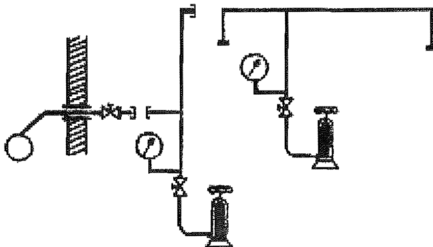
Εικόνα 8: Δοκιμή Αντοχής
