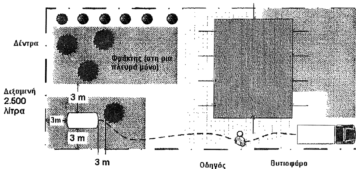
Σχεδιάγραμμα 2: Δεξαμενή σε μικρό υποστατικό
