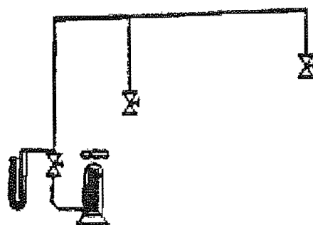
Εικόνα 9: Δοκιμή Στεγανότητας
